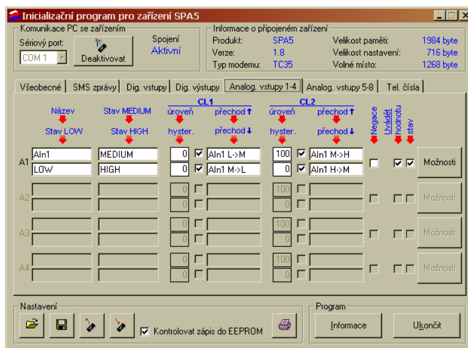
Obrázek 23 – Panel „Analogové vstupy“
