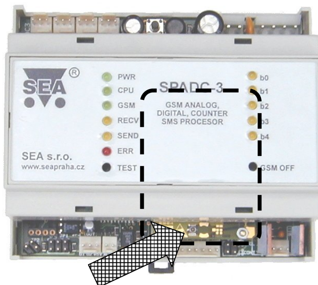
Obrázek 39 – GSM modem a pozice anténního konektoru
