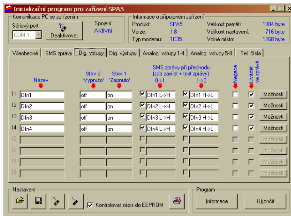
Obrázek 19 – Panel „Digitální vstupy“
