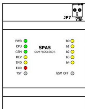
Obrázek 31 – Umístění konektoru JP7 (Napájení)
