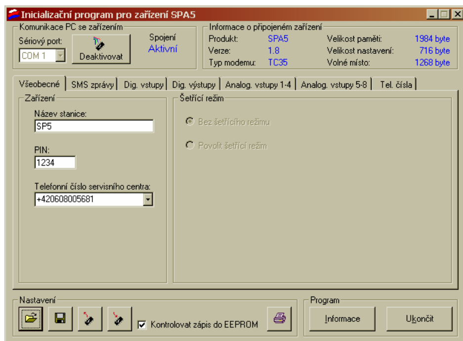
Obrázek 17 – Panel „Všeobecné“
