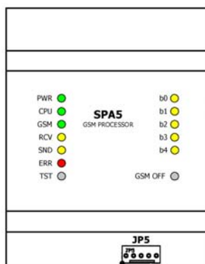
Obrázek 33 – Umístění konektoru JP5 (Digitální vstupy)
