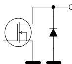
Obrázek 37 – Vnitřní zapojení digitálních výstupů O1 a O2
