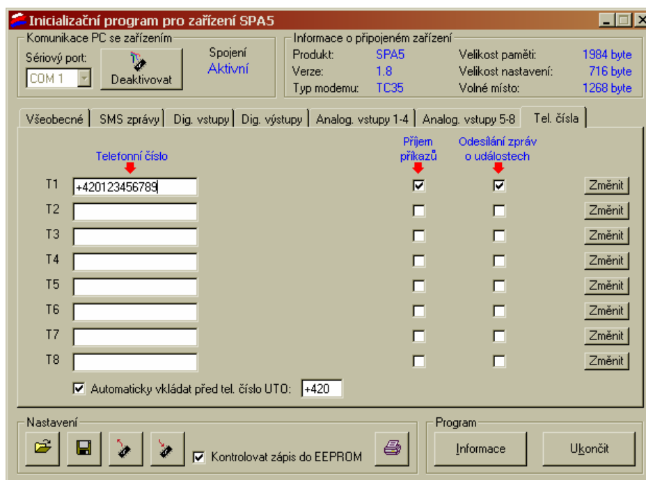
Obrázek 26 – Panel „Telefonní čísla“
