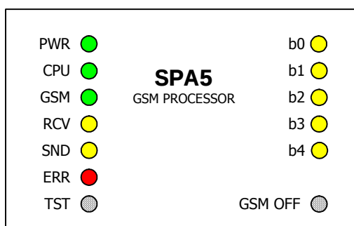
Obrázek 42 – Horní panel zařízení
