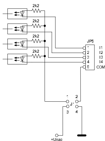
Obrázek 34 – Zapojení digitálních vstupů
